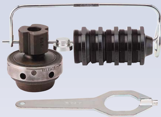
E Mandrin à mamelon
